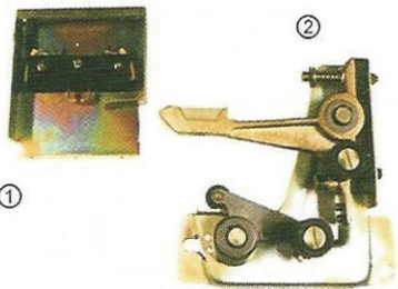
Interlock
