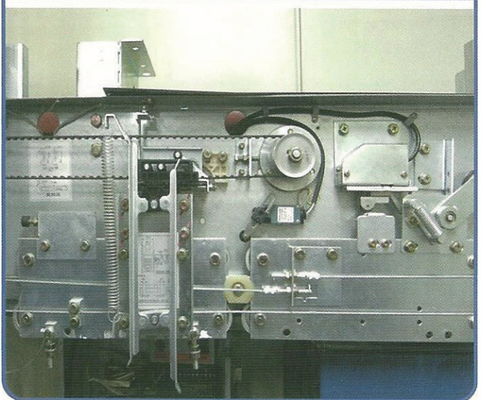
Hatch Door Hanger 058
