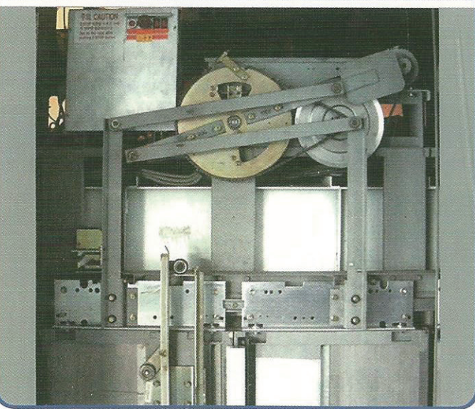
Hatch Door Hanger 057
