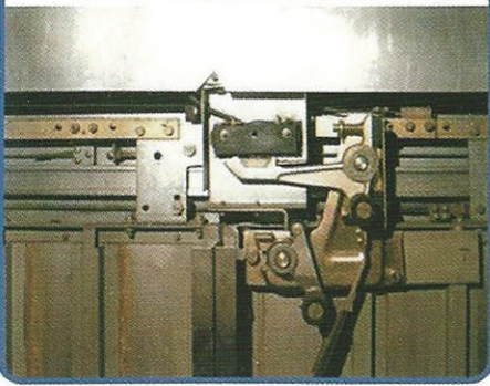
Hatch Door Hanger 063
